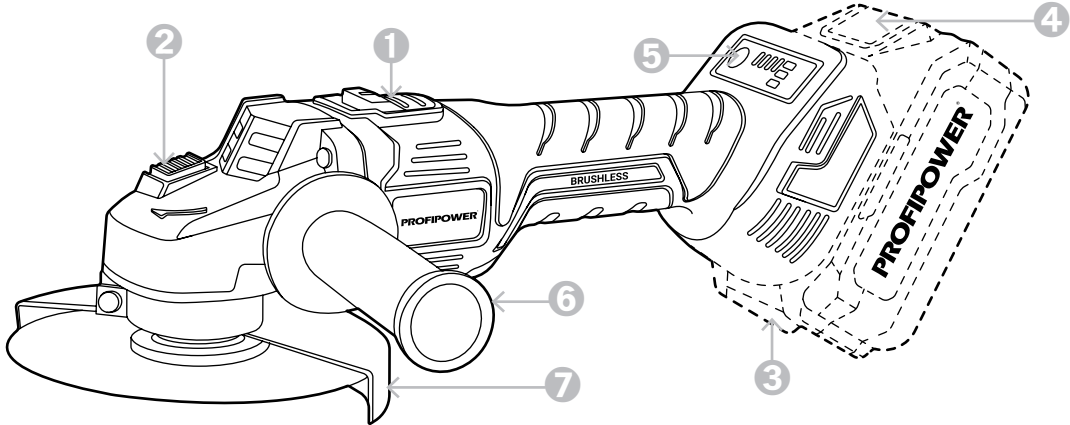
Рисунок 1.4.1. Устройство инструмента
