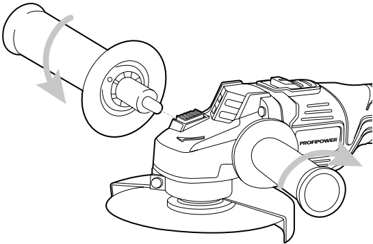
Рисунок 2.2.3. Установка боковой рукоятки
